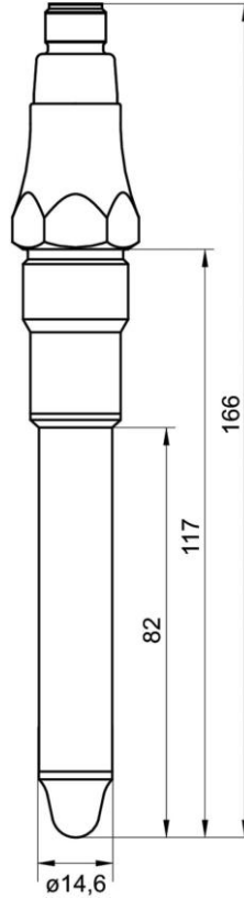
G 1/2 A гигиеническое, длина 82 мм (BCID: A03)
